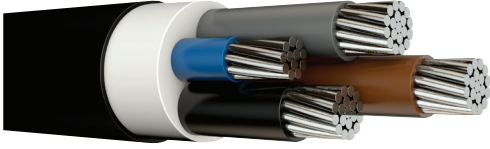
0,6/1 kV NAYY (YAVV) Tek veya Çok Damarlı Enerji Kablosu, Alüminyum İletkenli, PVC İzoleli, PVC Kılıflı
